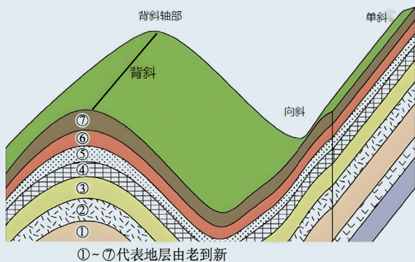
图一 地层结构 (作者供图)
