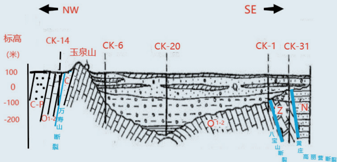
图二 玉泉山和昆明湖凹陷地质剖面图（作者供图）
