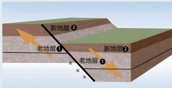
图三 断裂带两侧示意图（作者供图）
