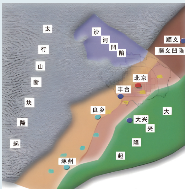
图四 北京地区燕山运动后古地形示意图 (作者供图)
