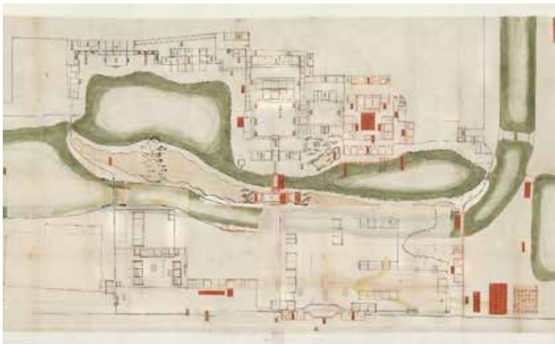
《新拟地盘画样》(118-0030) (作者供图)
